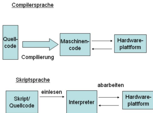
Bild 0-1: Unterschied zwischen Compiler- und Skriptsprache
